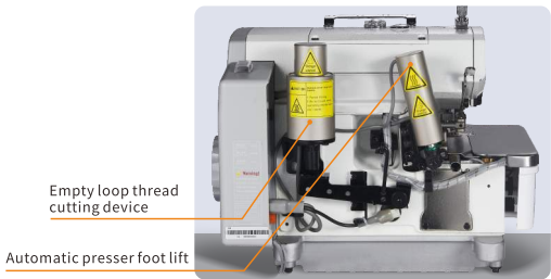
空环切线装置 (电磁铁式样) Empty loop thread cutting device (electromagnet style) 自动抬压脚 (电磁铁式样) Automatic presser foot lift (electromagnet style)
