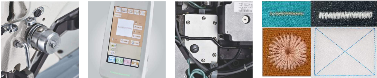
电子夹线 Electronic thread clamp 可选配液晶屏面板 Optional LCD panel 全封闭下轴齿轮超耐磨 super durable closed bottom shaft gear
