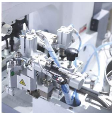
气动送扣系统 Pneumatic button feeding system
