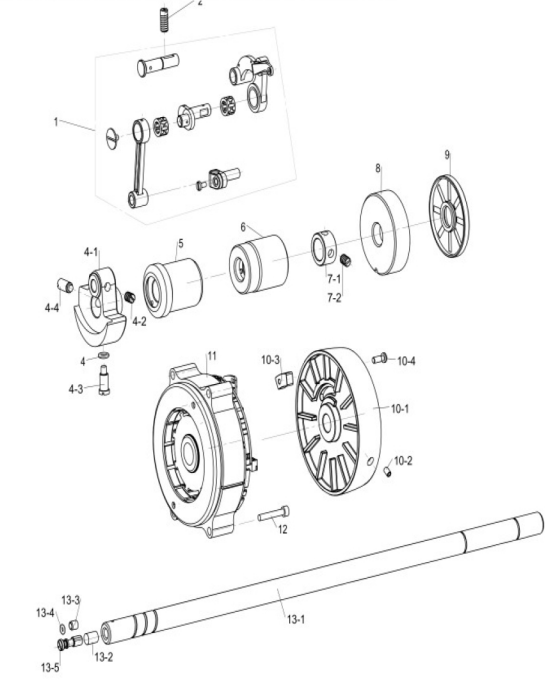
2. 上盖、挑线装置 / MAIN SHAFTHREAD-UP LEVER MECHANISM
