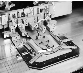
普通换模贴袋机 正常换一套模具安装调试需6-8小时。
