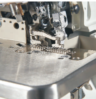
上下差动牙 top differential feed dog.
