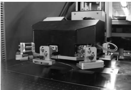
PK 快速换模贴袋机 三分钟轻松解决换模问题，无需任何调试。
