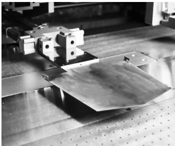
普通换模贴袋机 正常换一套模具安装调试需6-8小时。
