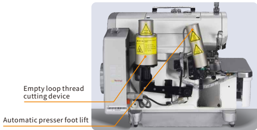
空环切线装置 (电磁铁式样) 自动抬压脚 (电磁铁式样) Empty loop thread cutting device (electromagnet style) Automatic presser foot lift (electromagnet style)
